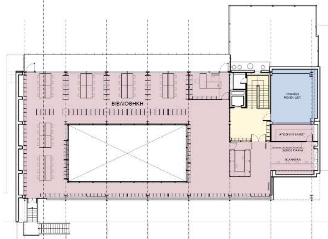
0.4 Κάτοψη Ορόφου Σ5 (Βιβλιοθήκη)
