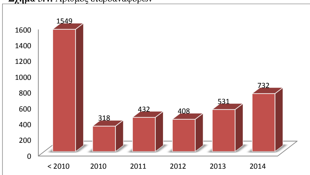
Σχήμα 5.4: Αριθμός ετεροαναφορών*
